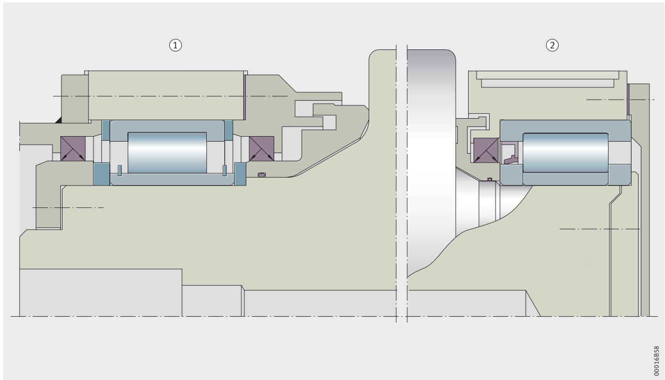
图 2 · 导辊采用的轴承布置 ① 浮动端, ② 固定端
